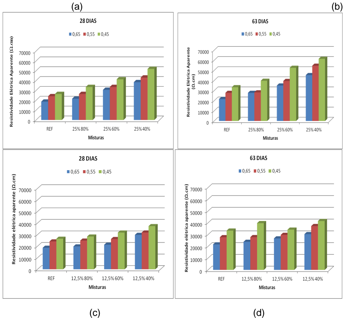
Figura 30 - Valores de resistividade elétrica aparente em função da relação a/c (a) 25% AMRC aos 28 dias, (b) 25% AMRC aos 63 dias, (c) 12,5% AMRC aos 28 dias, (d) 12,5% AMRC aos 63 dias.
