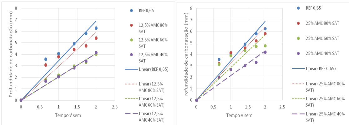
Figura 24 - Linhas de tendência para as misturas de referência e com substituição de 12,5% e 25% de AMRC, para relação a/c=0,65.
